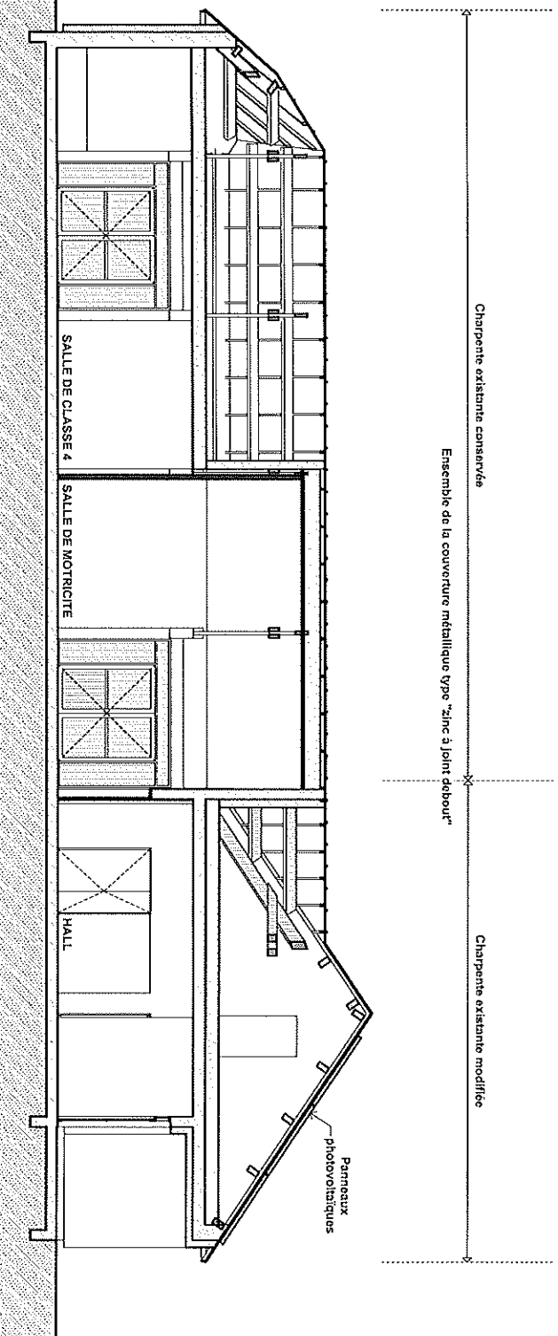
COUPE A
